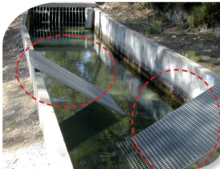
Exemple d'échelles fixées sur bajoyers inclinés ou verticaux afin d'aider les animaux à s'extraire du canal.
